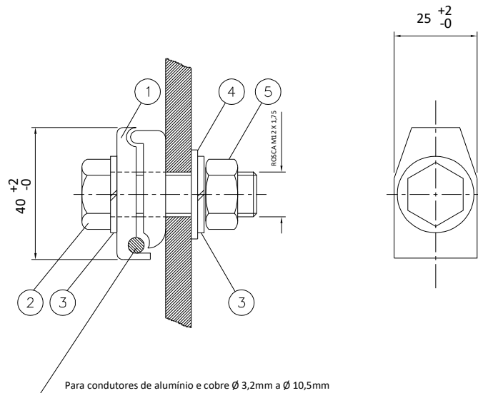
Figura 4 – Conector de Aterramento
