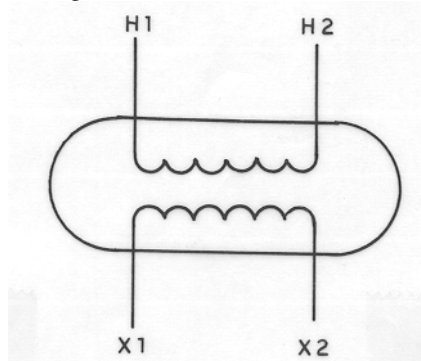
Figura 6 – Polaridade Subtrativa
