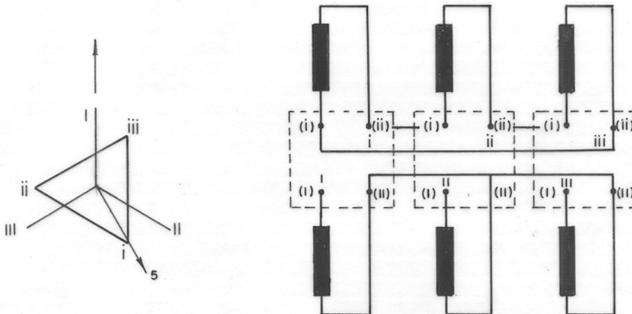
Figura 7 – Exemplo de 3 Transformadores Monofásicos Ligados para Formarem um Banco Trifásico (Designação Yd5)
