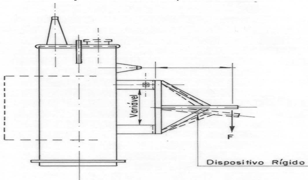
Figura 5 – Detalhe do Ensaio de Suportabilidade Mecânica
