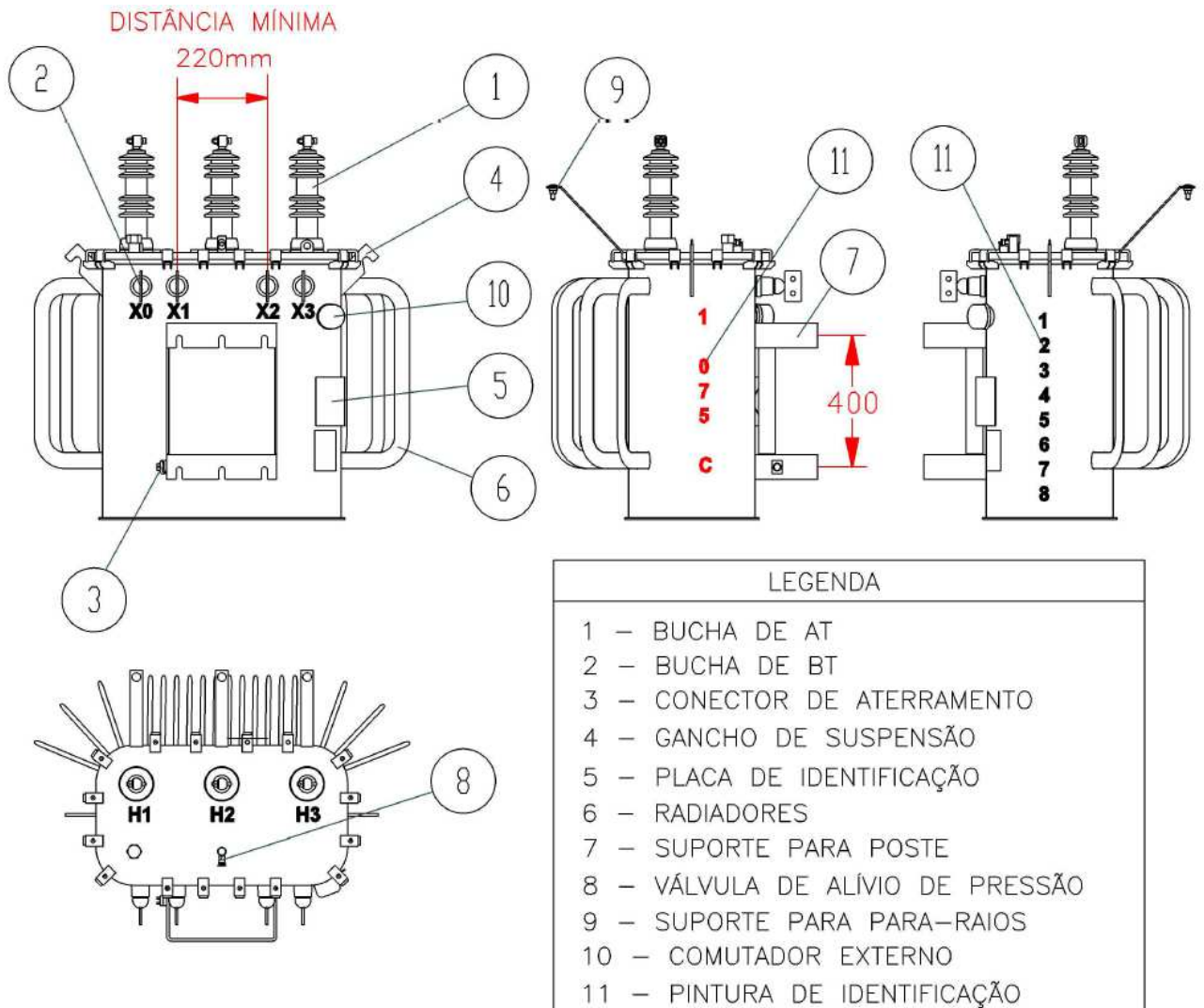
Figura 2 – Transformadores Trifásicos
