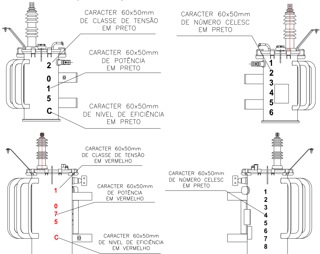
Figura 3 – Exemplos de Pinturas de Identificação
