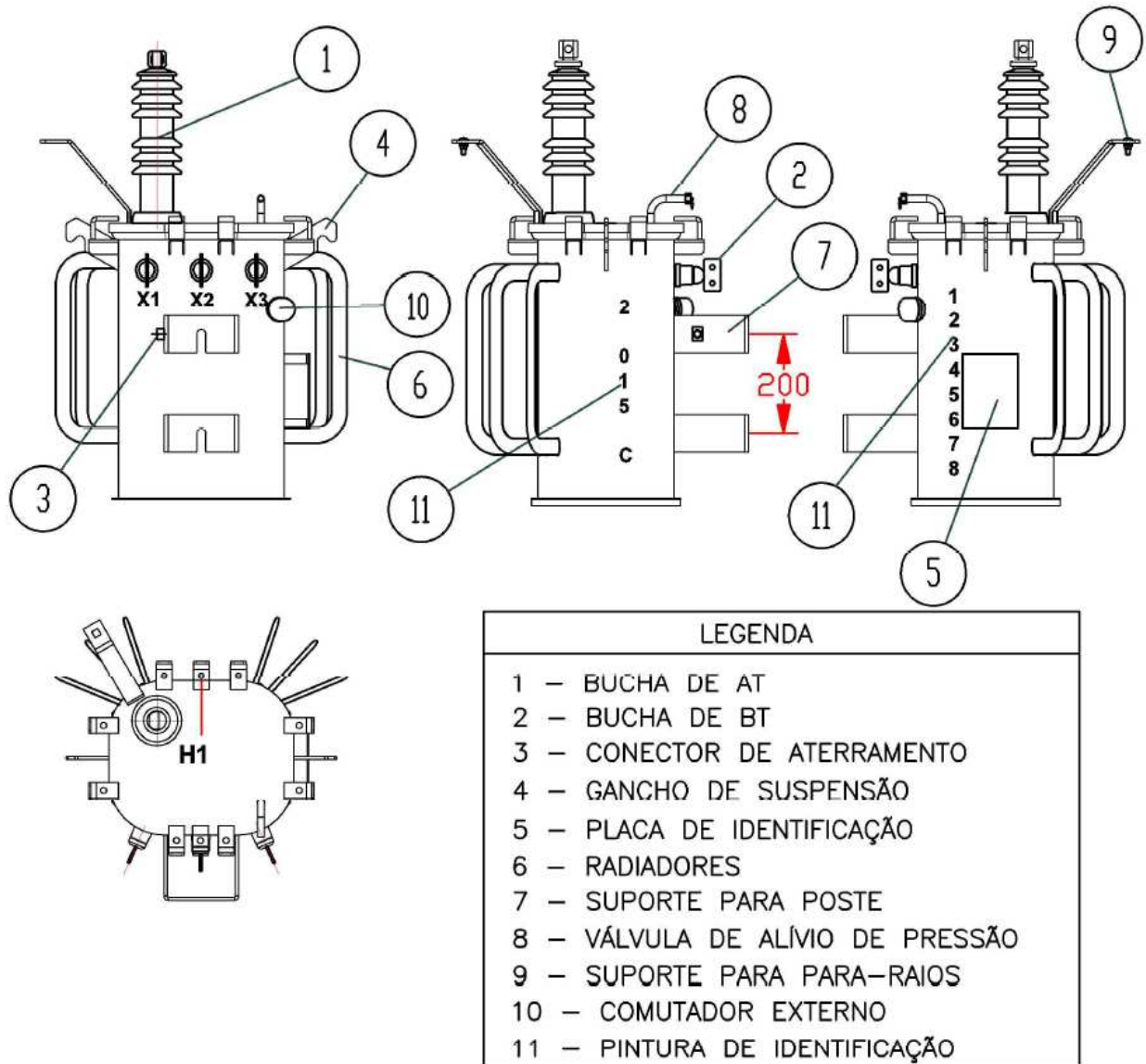
Figura 1 – Transformadores Monofásicos
